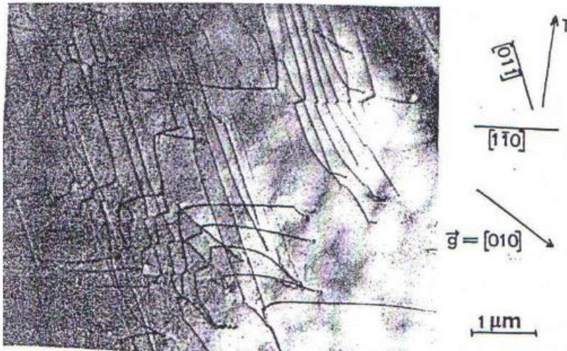
Fig. 4: Observation des dislocations dans un microscope électronique classique. Dû au contraste de diffraction, les dislocations apparaissent sous forme de lignes noires. Echantillon Aluminium, Photo M. Carrard, Thèse EPFL 1985 (Agrand. 15 000 x)
